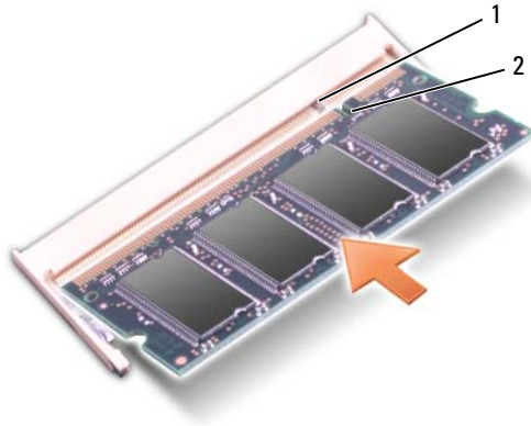
1 Klammer 2 Kerbe
