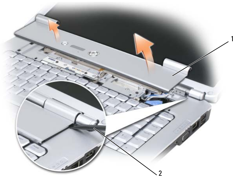
1 Scharnierabdeckung 2 Stift
