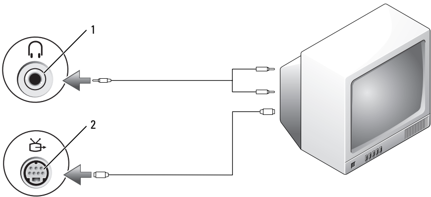
1 Audioanschluss 2 S-Video-TV-Ausgang
